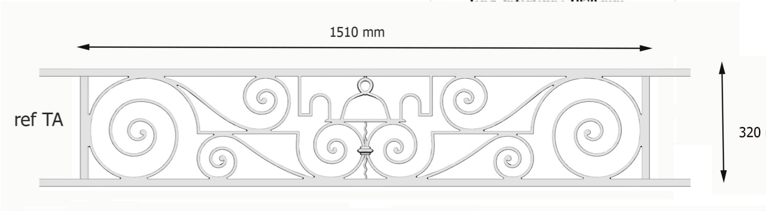
RG haut : 800 mm long hors tout : 1270 mm long intérieur : 1070 mm
