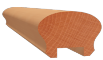
Pasamanos de madera - LO580 34 x 50 mm
